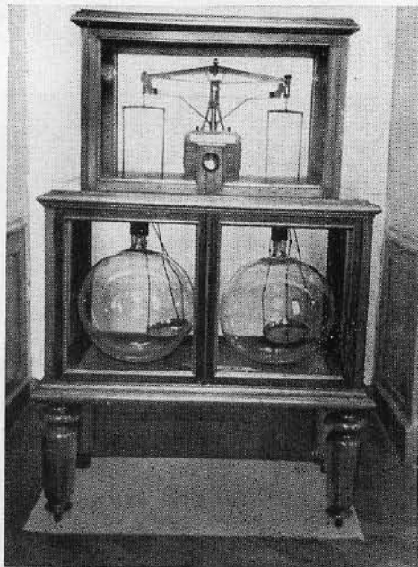
Двухъярусные весы Менделеева для взвешивания газов. 1870.
